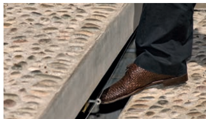
01 H Unterhalb des sich komplett absenkenden Deckels der Anlage ist ein umlaufendes Sicherheitsseil. Wird es betätigt, stoppt die Anlage sofort. A safety cable runs below the lid of the unit. Once touched, the system stops immediately.
